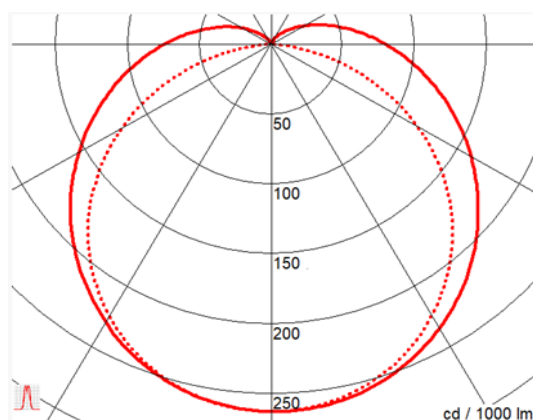
Courbe photométrique
