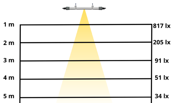
Échelle d'intensité
